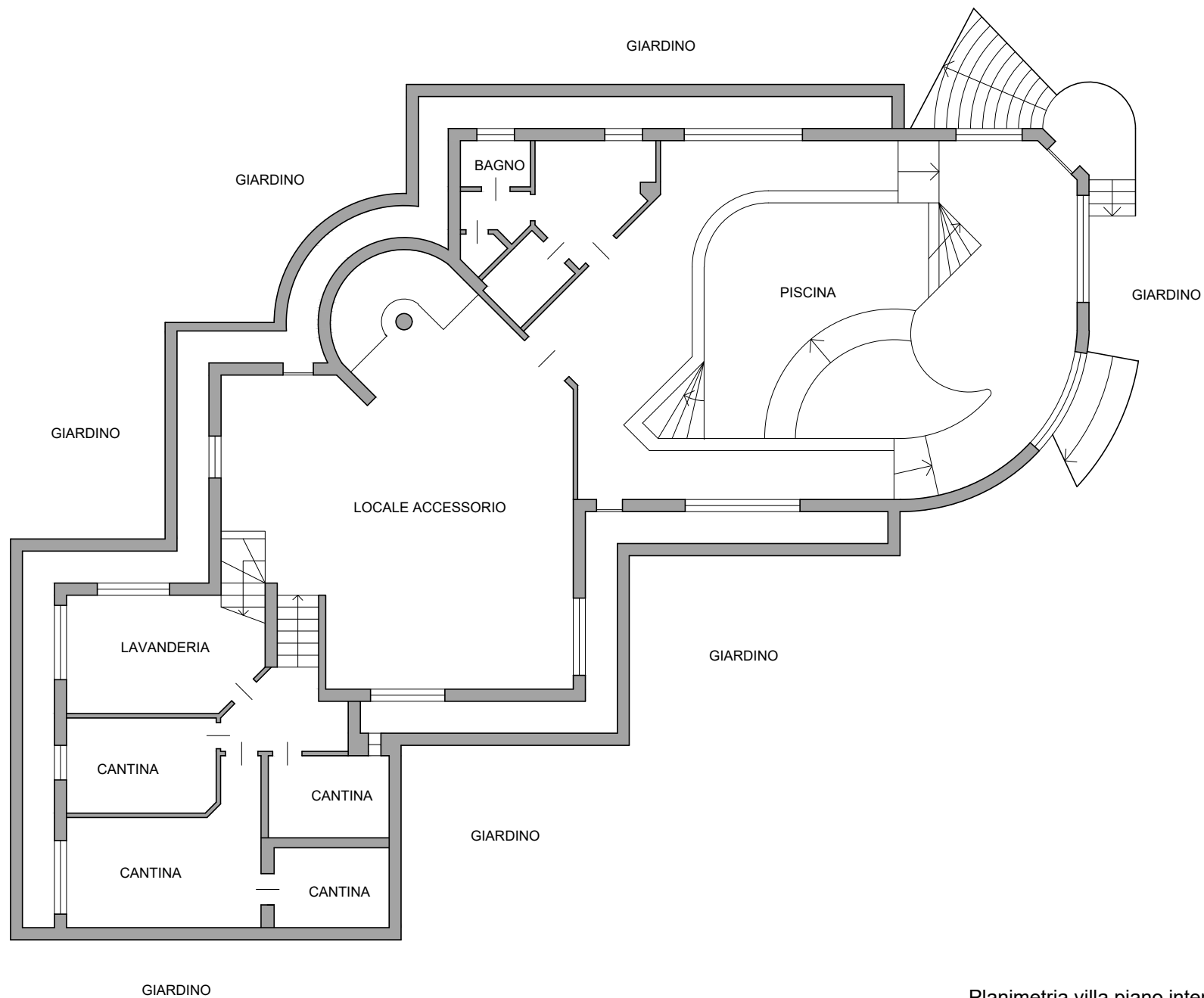
Planimetria villa piano interrato Via della Chiocciola n°32, Carimate (Co)
