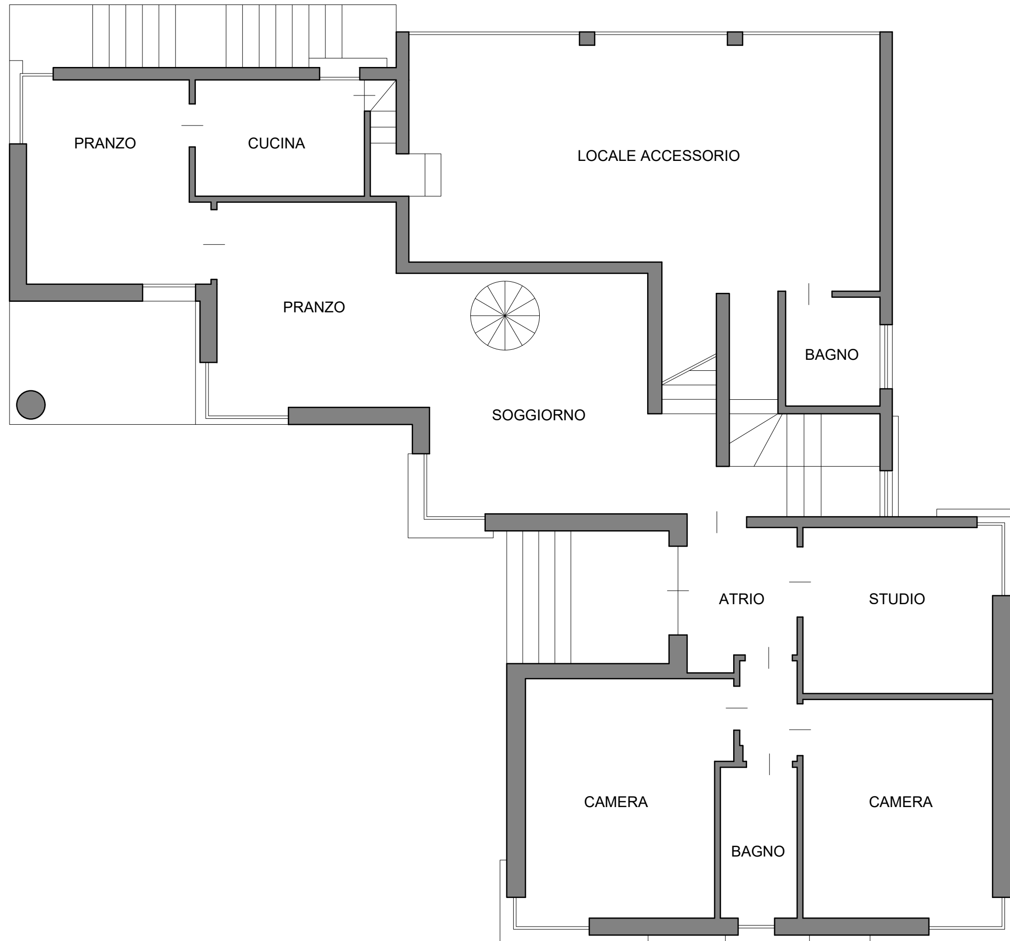
Planimetria villa _ piano rialzato Via Monte San Martino n.102, Gallarate (VA)
